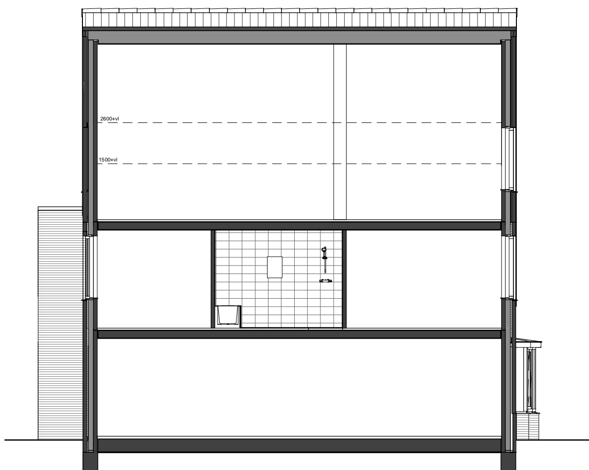
Doorsnede
