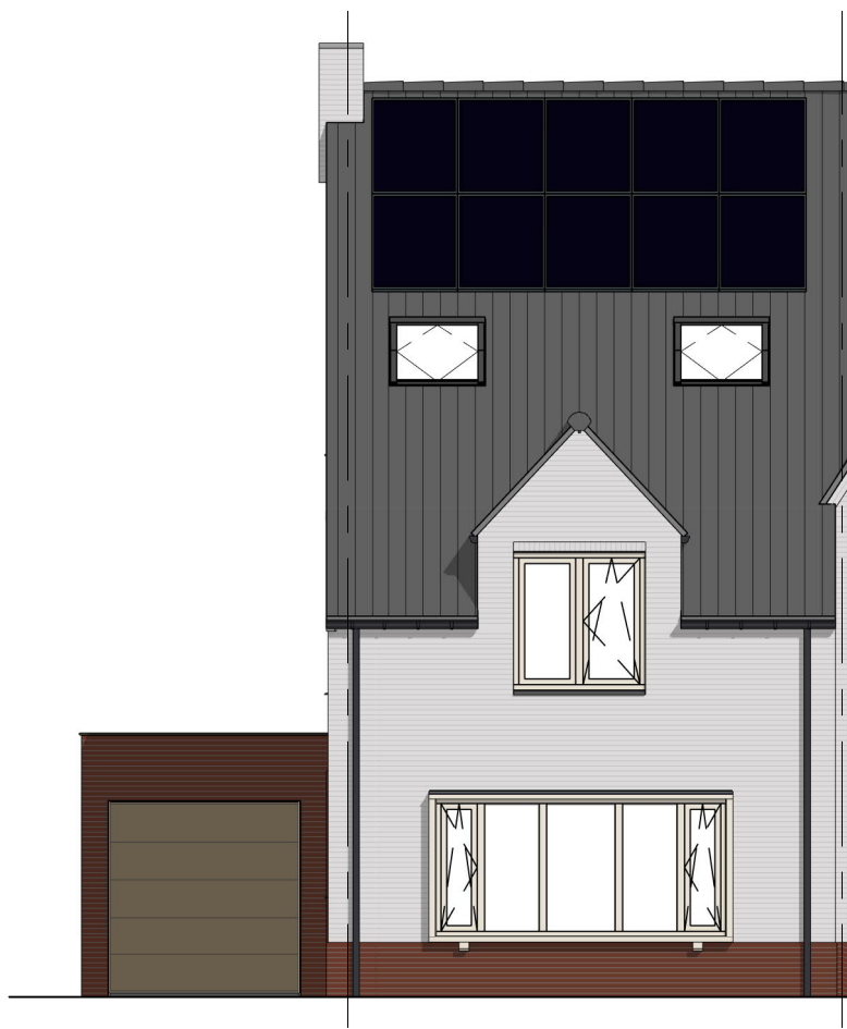
Vorgevel
