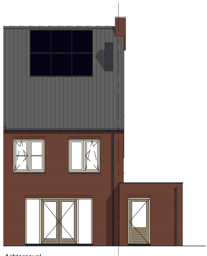
Achtergevel
