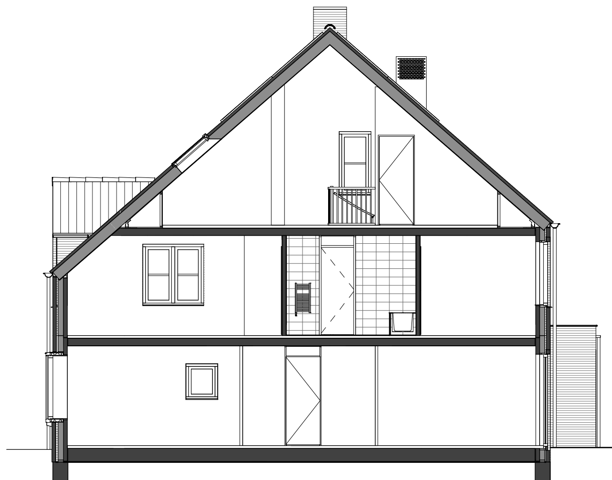
Doorsnede
