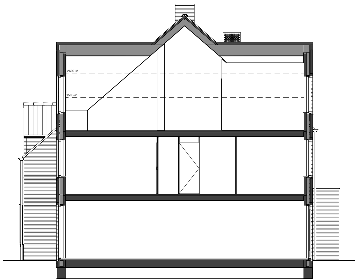
Doorsnede
