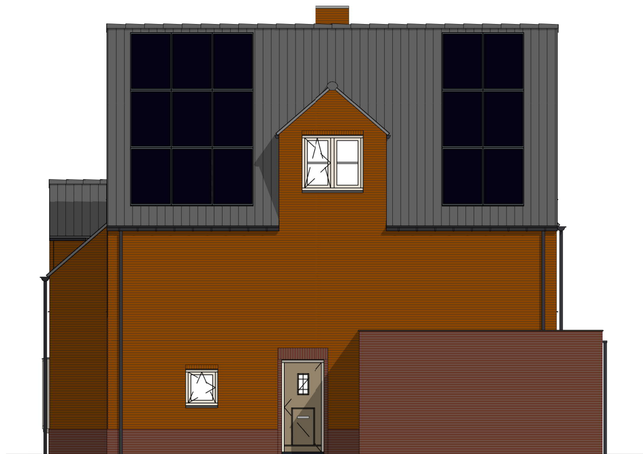
Zijgevel
