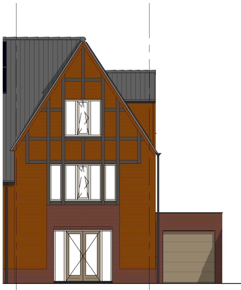
Voorgevel
