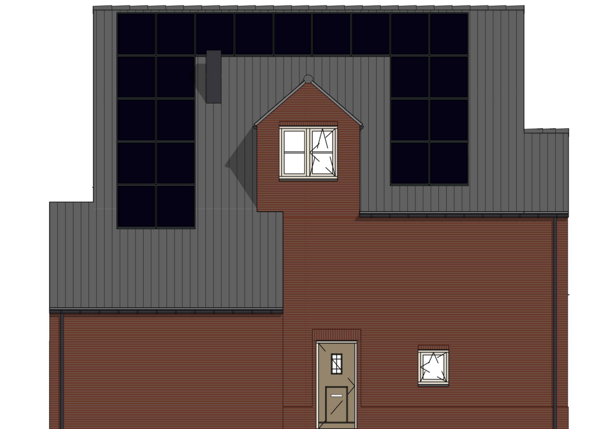
Zijgevel
