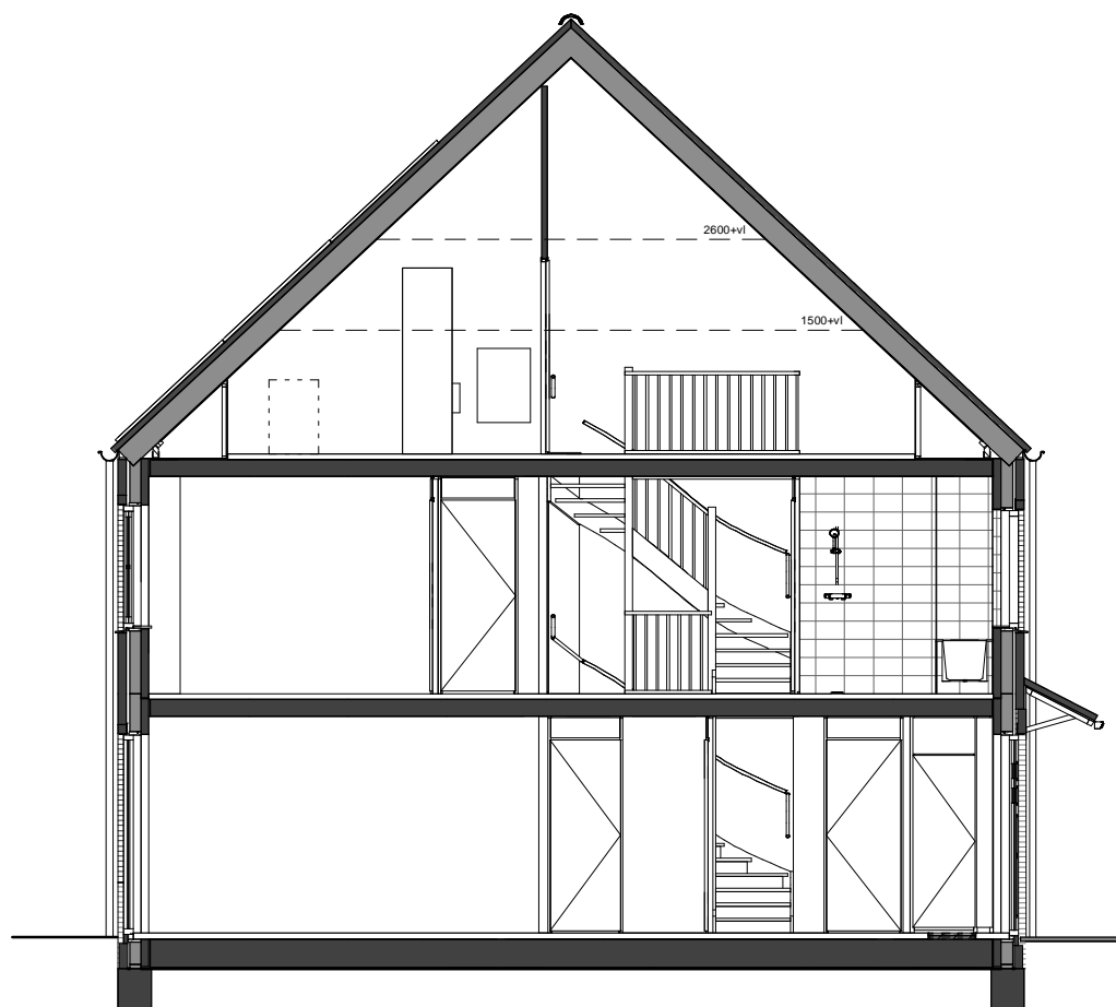
Doorsnede
