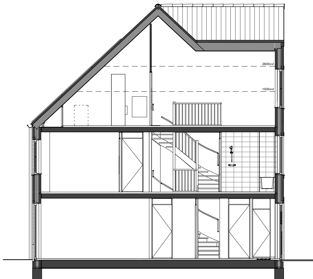
Doorsnede
