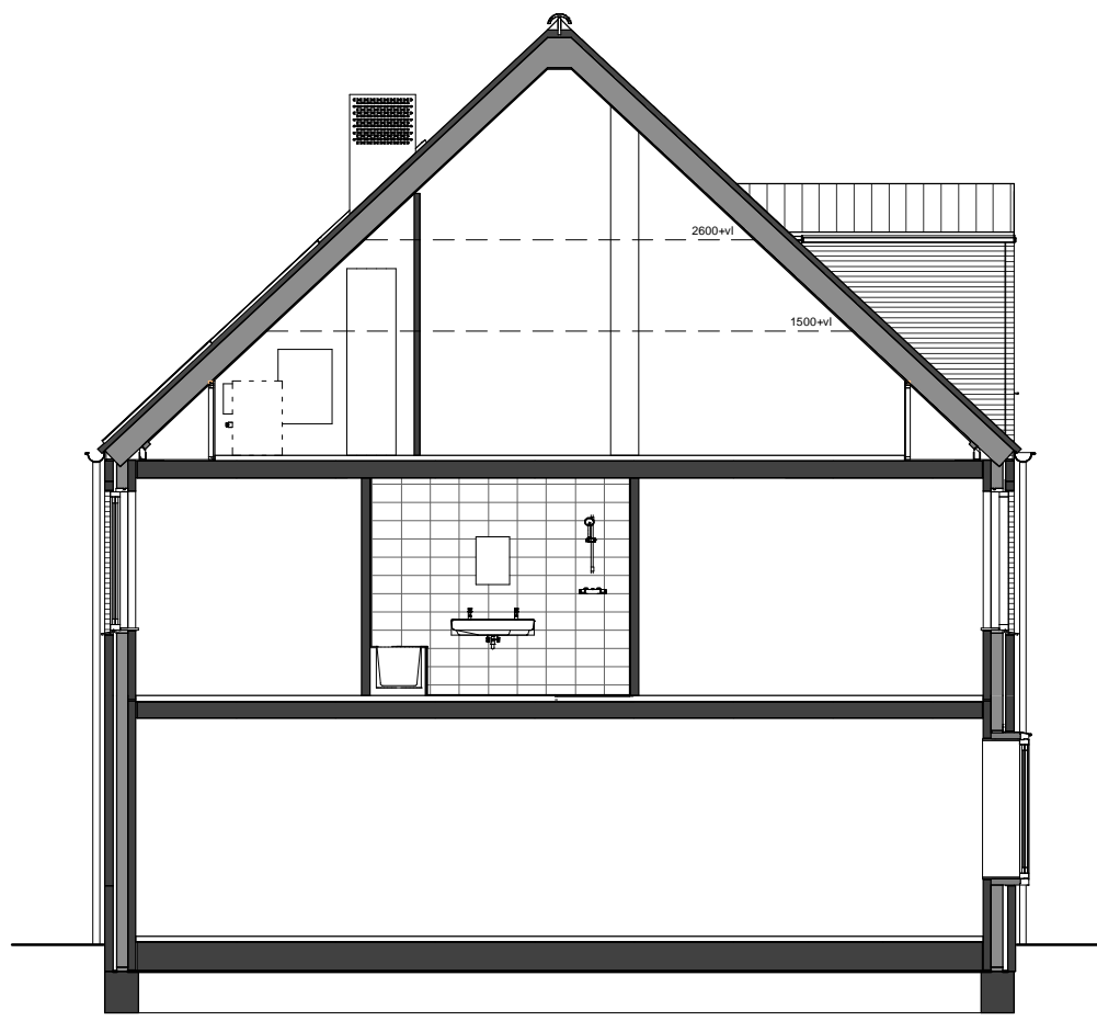
Doorsnede
