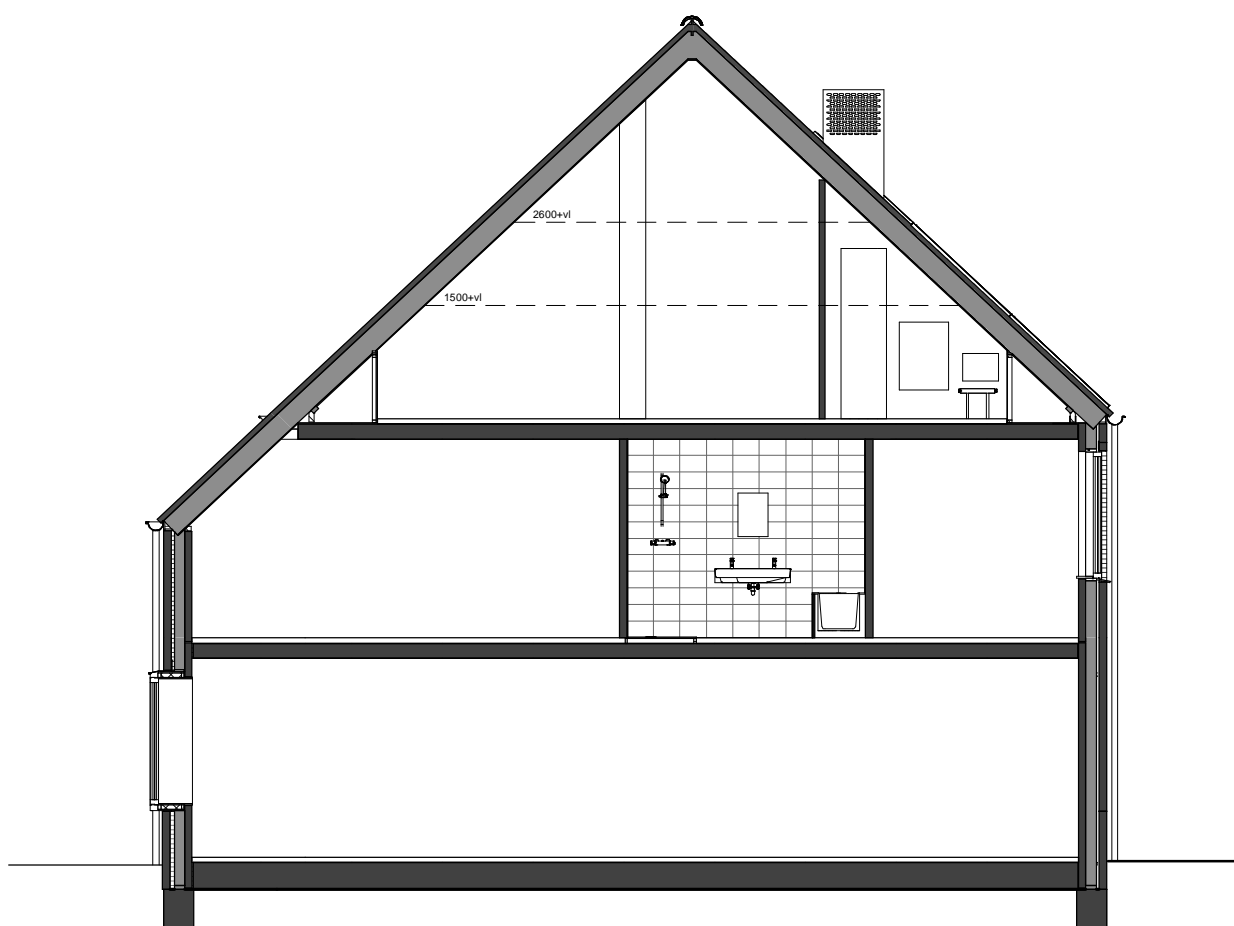
Doorsnede
