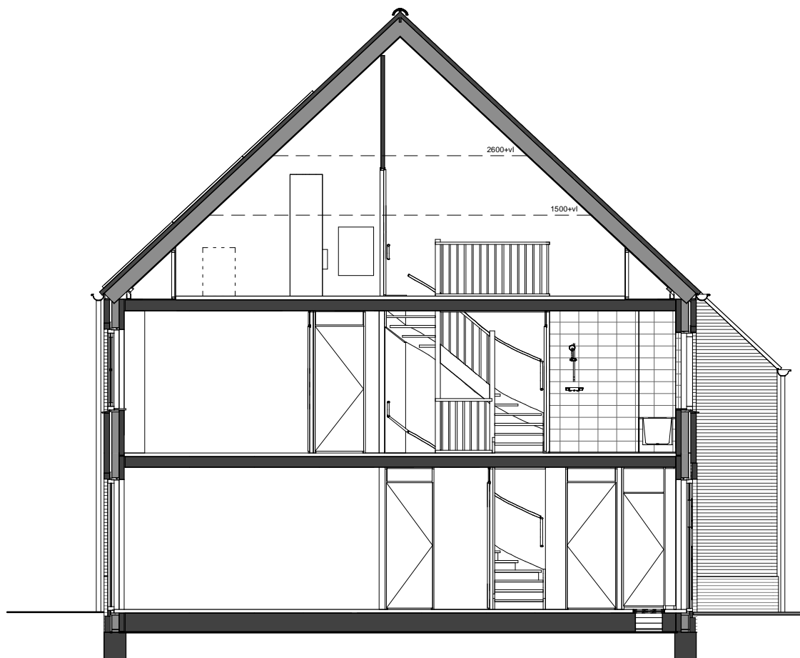
Doorsnede
