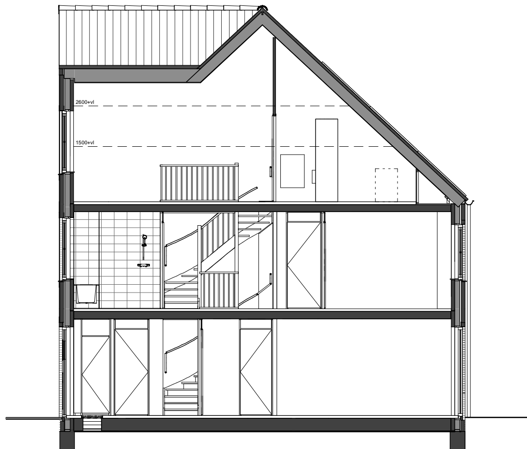
Doorsnede
