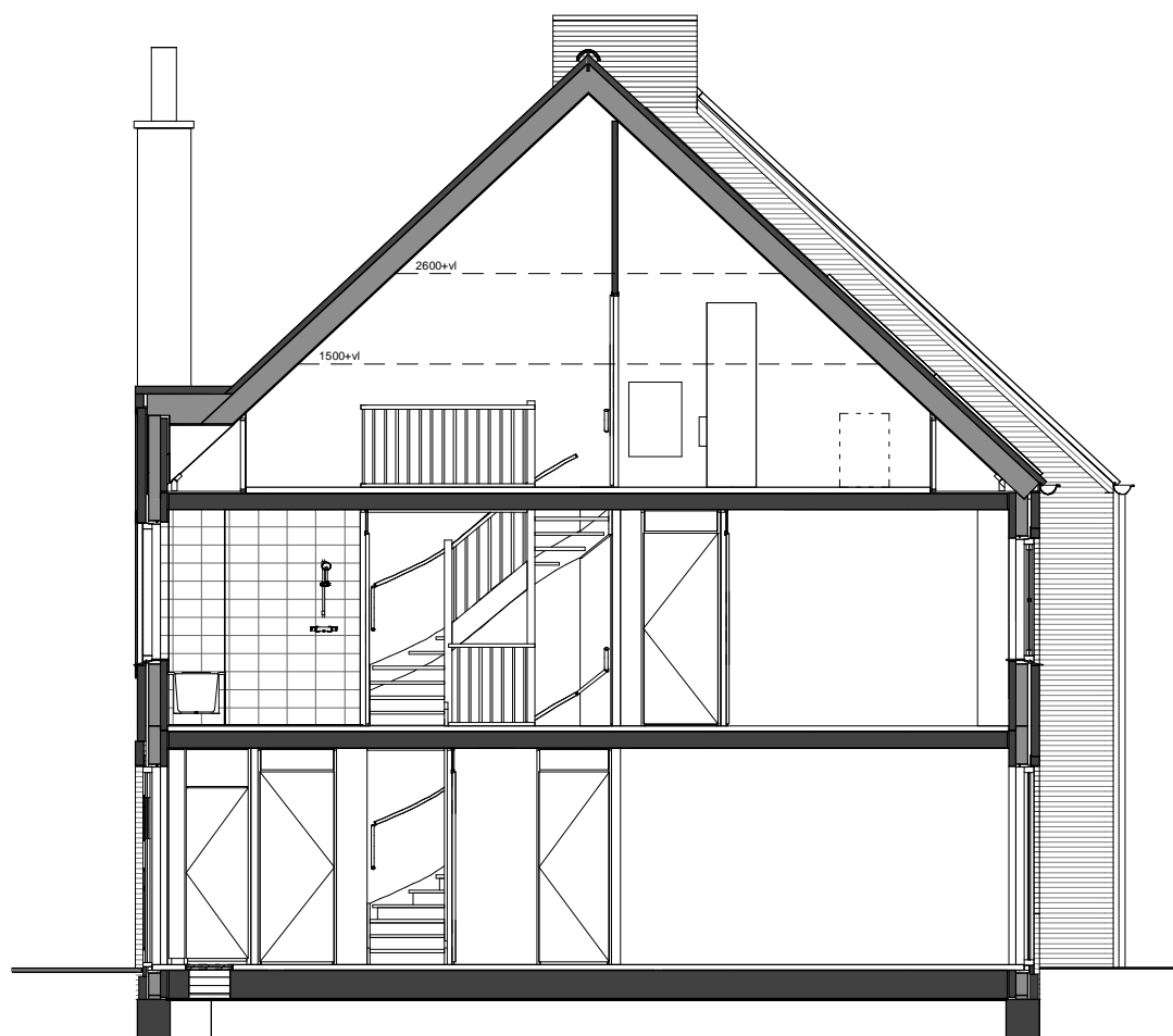
Doorsnede
