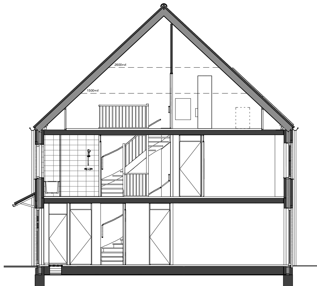
Doorsnede
