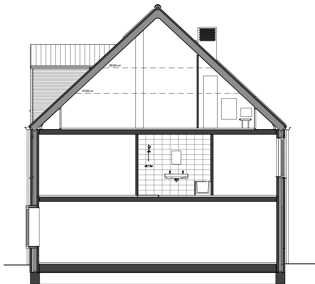
Doorsnede
