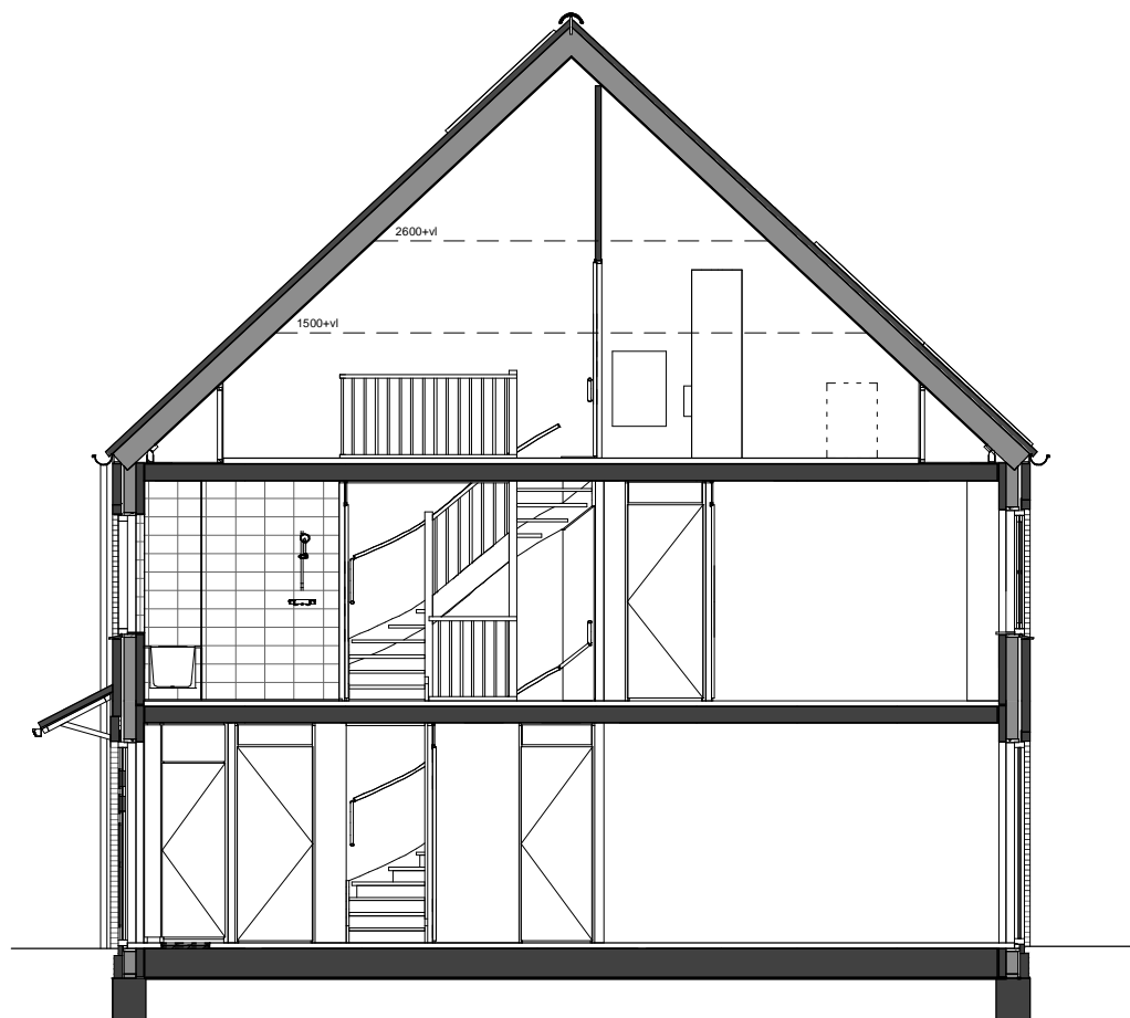
Doorsnede
