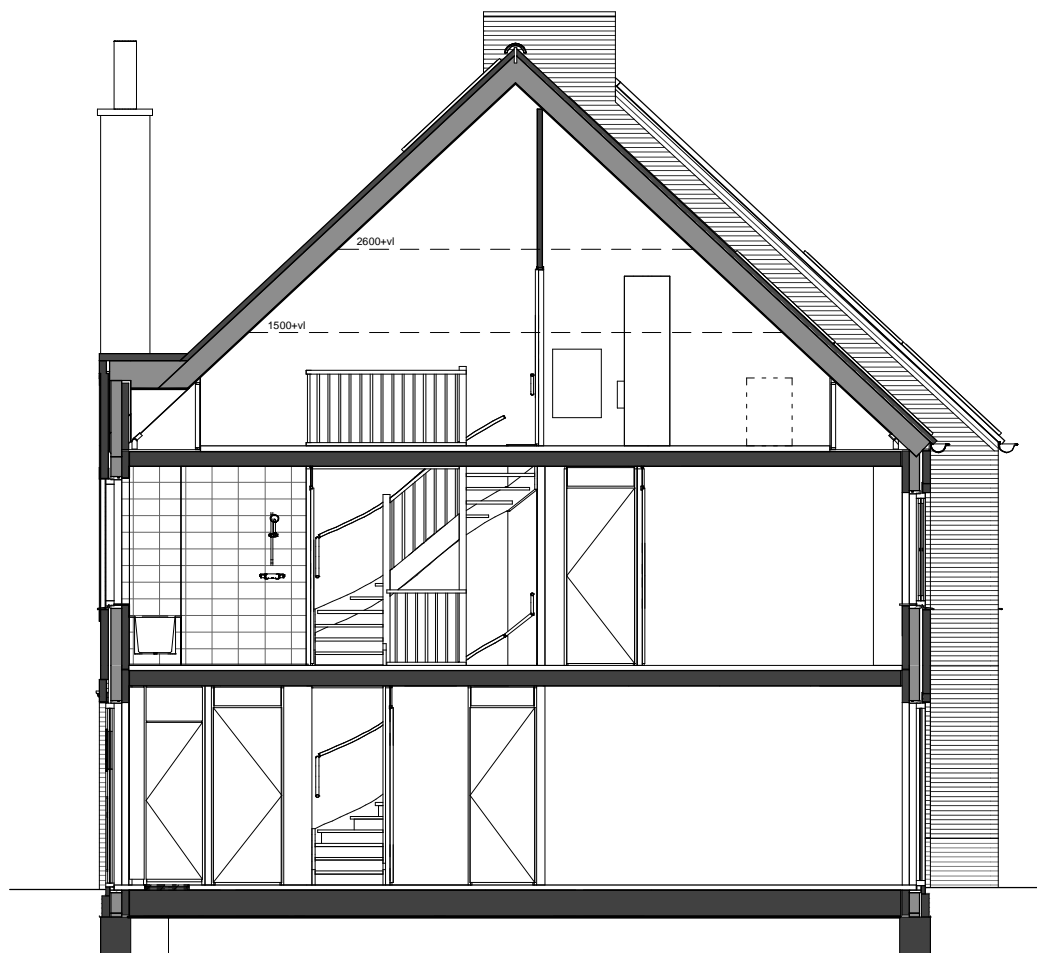
Doorsnede
