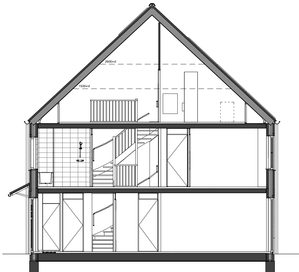
Doorsnede
