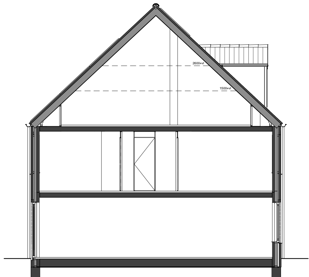
Doorsnede
