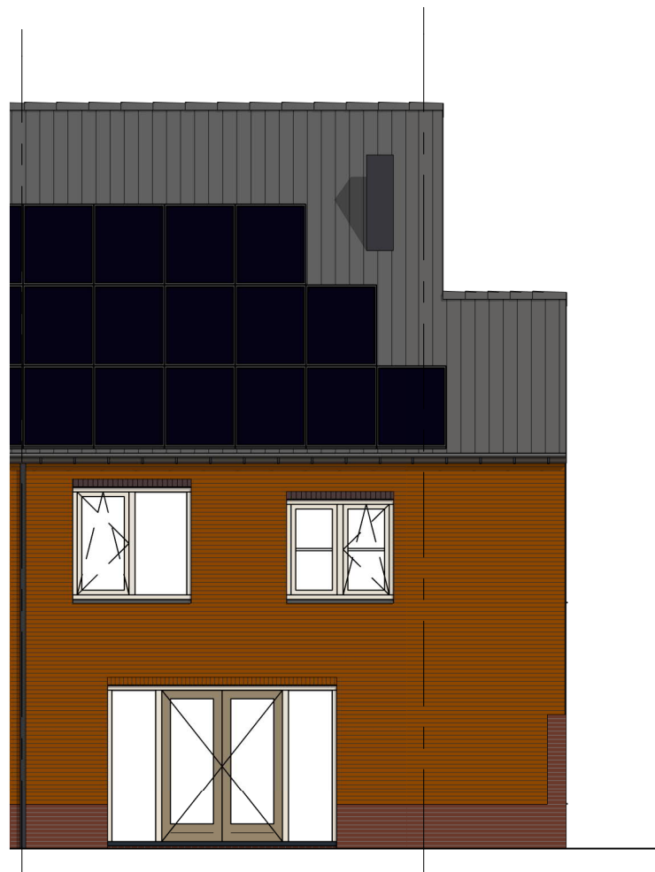
Achtergevel
