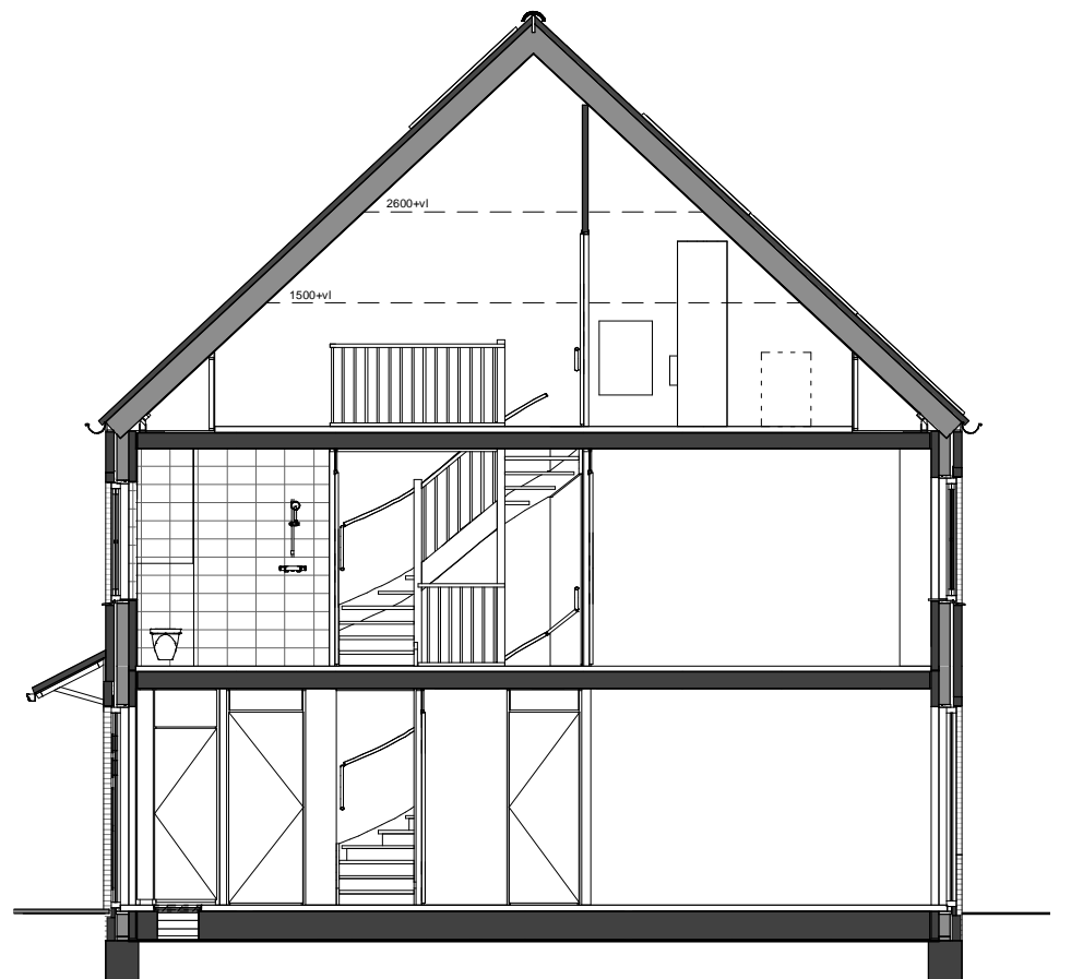
Doorsnede
