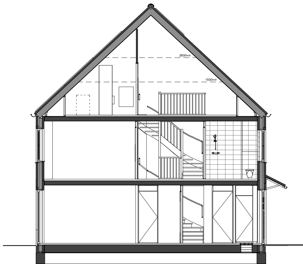
Doorsnede
