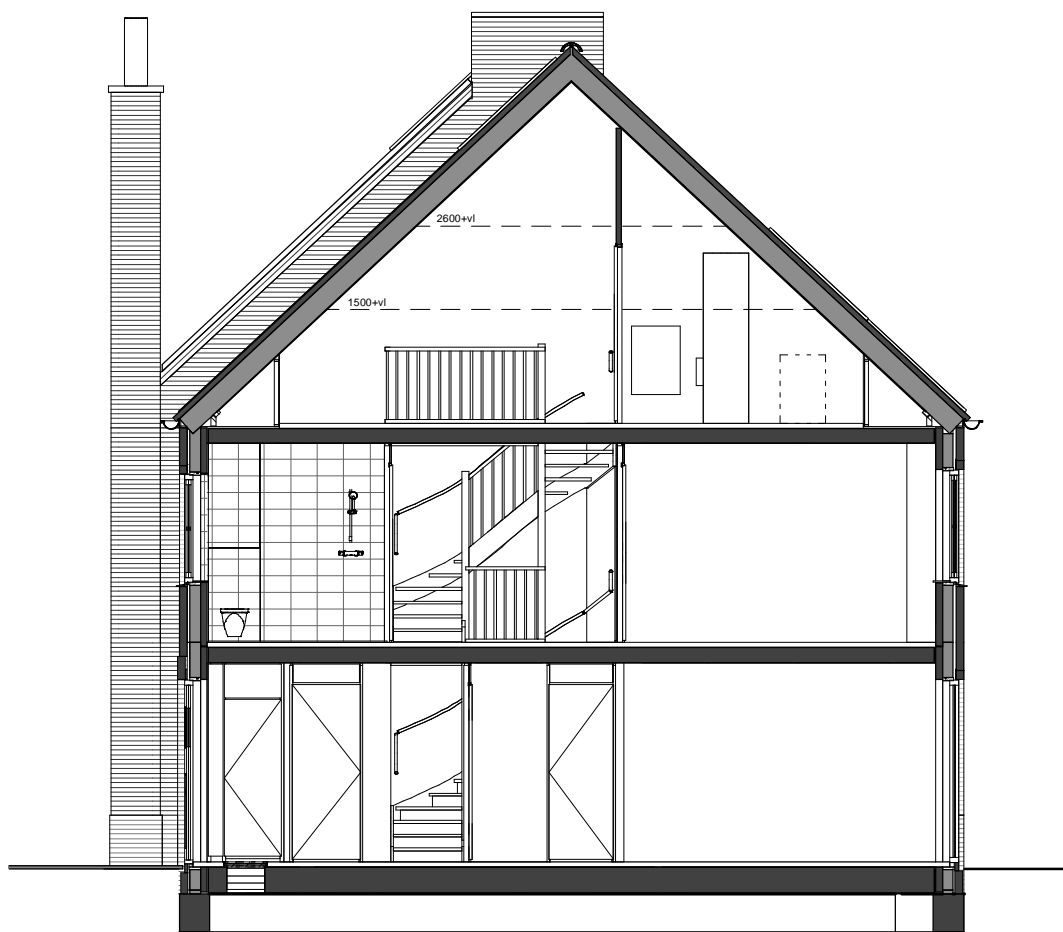
Doorsnede
