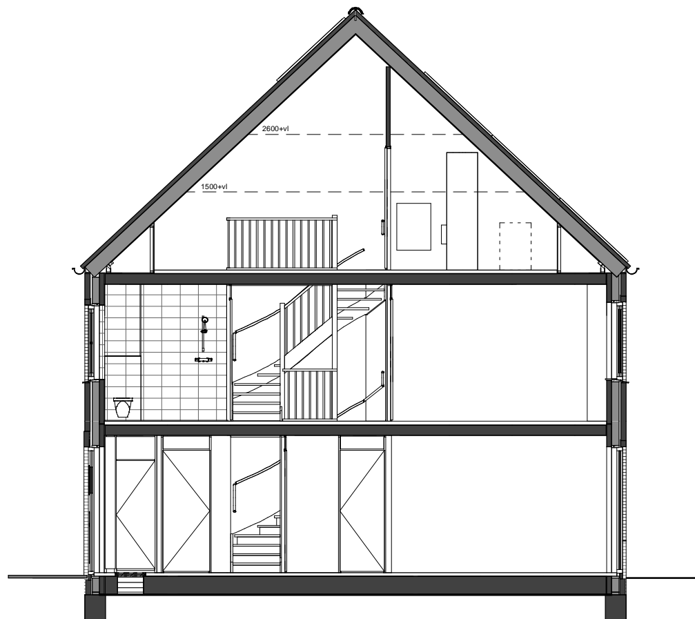
Doorsnede
