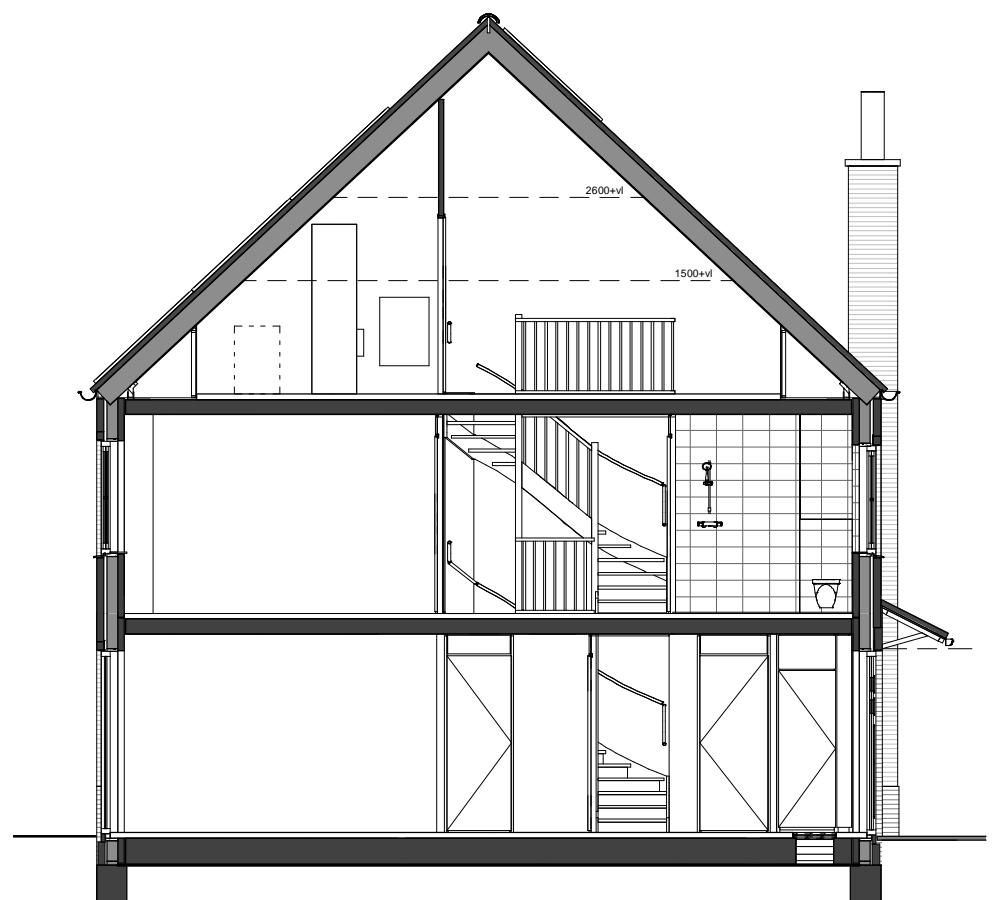
Doorsnede
